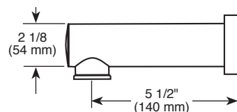
RP54874▲ (Pull-Down Diverter Tub Spout)
